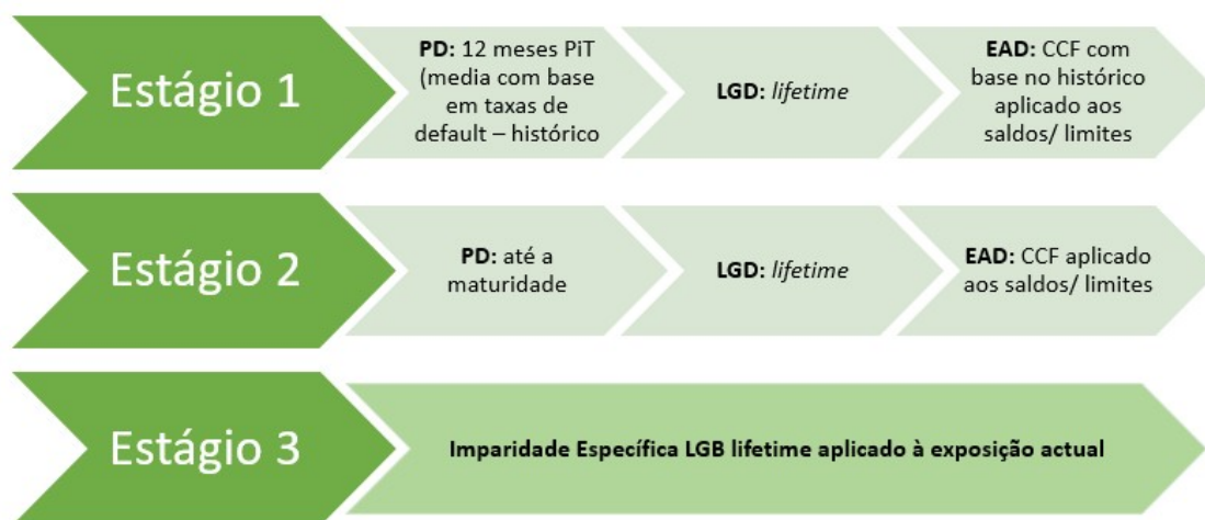
Figura 7: Elementos de cálculo da ECL
